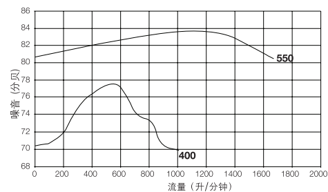
噪音级别
