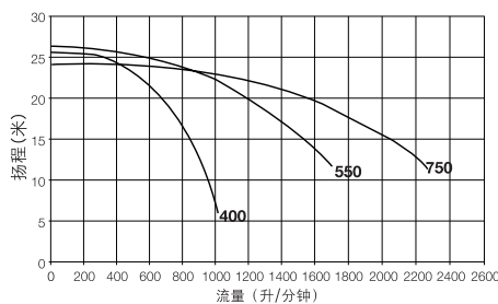
流量曲线
