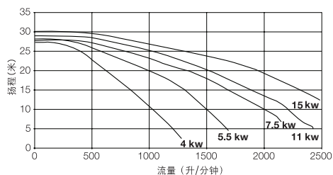
流量曲线
