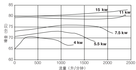
噪音级别
