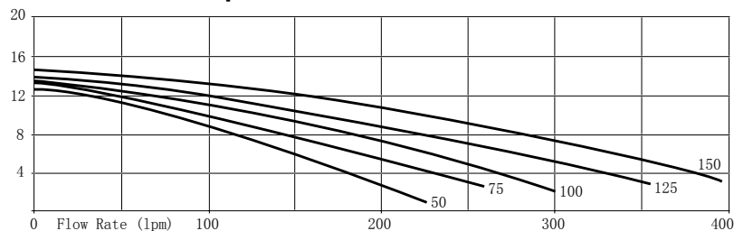
Aquastream太阳能水泵流量曲线
